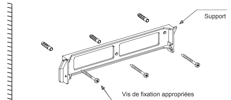
Figure 4.4 Montage mural de l'onduleur
