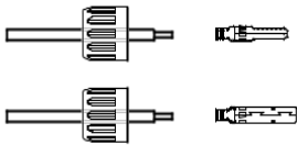
Figure 4.9 Insérez le fil dans le Connecteur Écrou borgne et broche de contact
