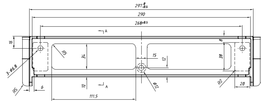
Figure 4.3 Montage mural de l'onduleur
