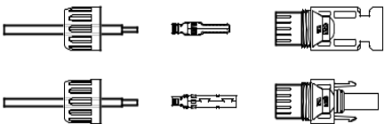
Figure 4.8 Démontage de l'écrou borgne du connecteur
