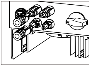
Figure 4.12 Connexion des connecteurs CC à l'onduleur
