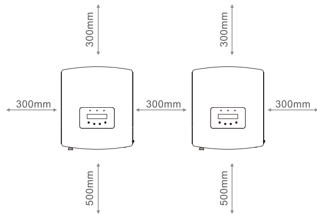
Figure 4.2 Espace libre pour le montage de l'onduleur
