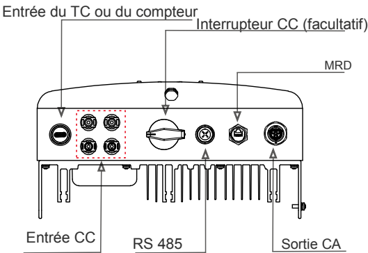
Figure 1.2 Vue latérale inférieure
