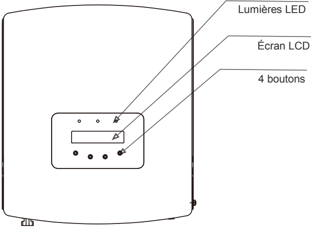
Figure 1.1 Vue de face
