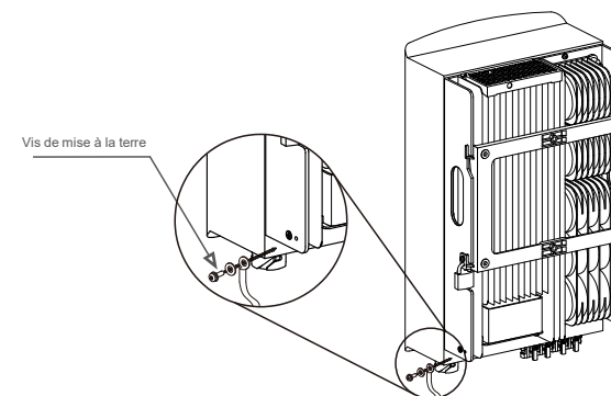
Figure 5.10 Câble fixé
