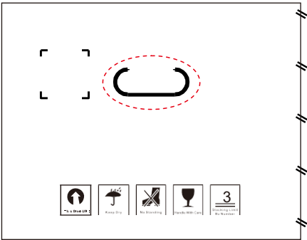
Figure 4.1 Déplacer l'onduleur
