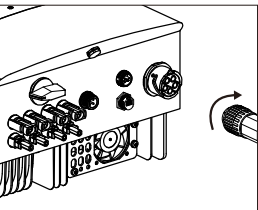
Figure 5.24 Connecteur CA vers l'onduleur
